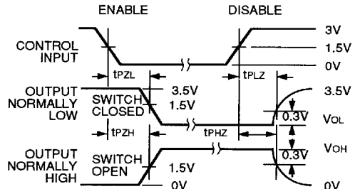
2567 drw 09
