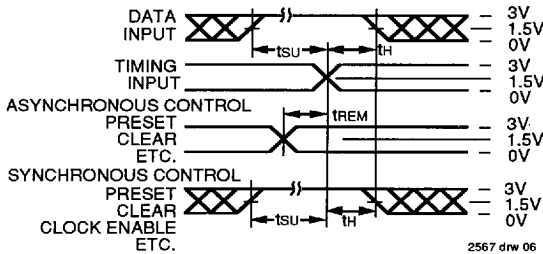
2567 drw 06
