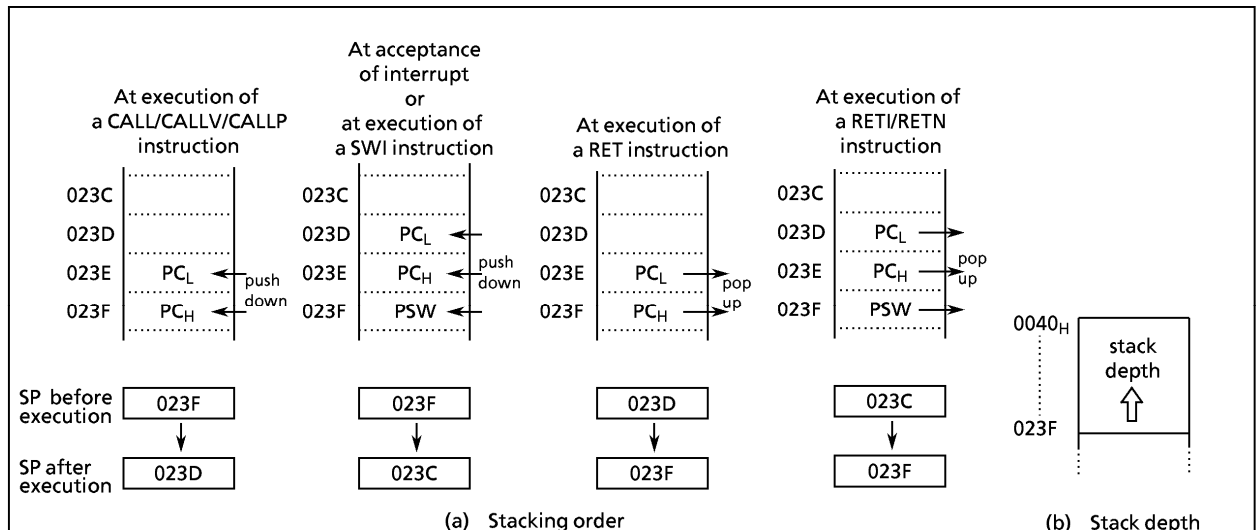
Figure 1-8. Stack
