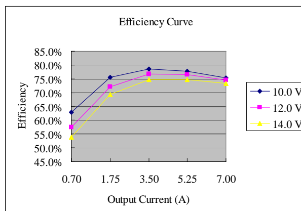
Vo=0.9 V
