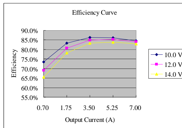
Vo=1.8 V
