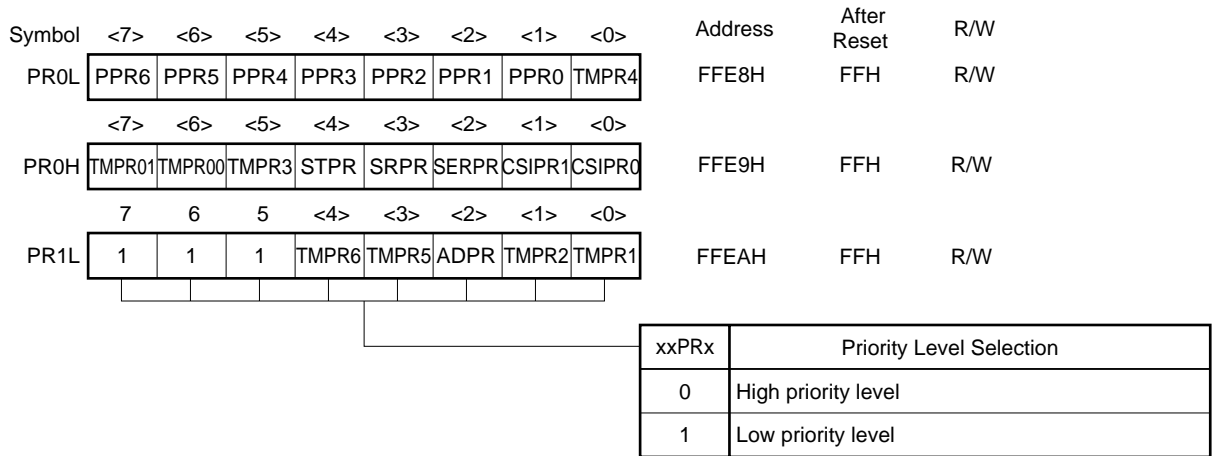
Figure 22-4. Priority Specify Flag Register Format
