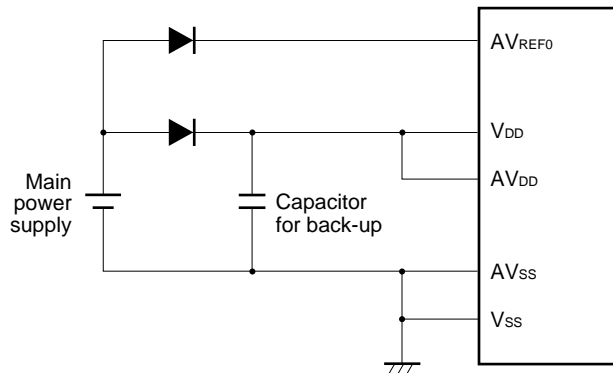
Figure 15-12. Handling of AV DD Pin
