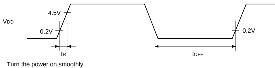
Fig. 9. Power-on reset
