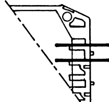
G 28 serie 110 (2,8 x 0,8 mm)
