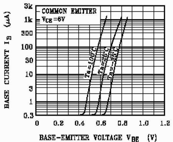
I_B - V_{BE}
