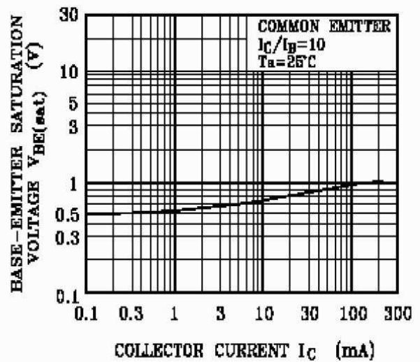
V_{BE(sat)} - I_C
