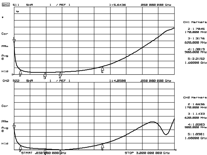
VSWRi, VSWRo
