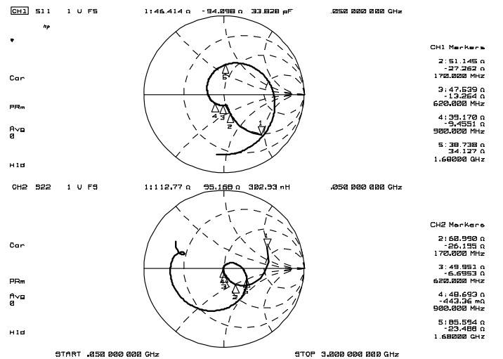
Zin, Zout
