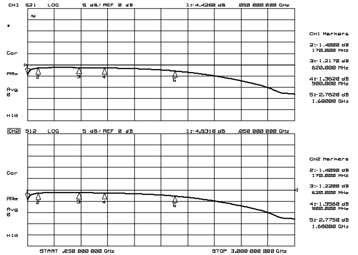
S21, S12
