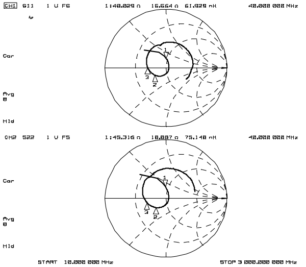
Zin, Zout (f=10MHz~3GHz)
