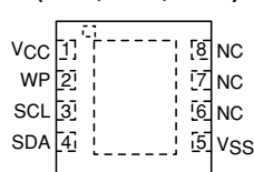
TDFN Package (RD4, ZD4, GD4)
