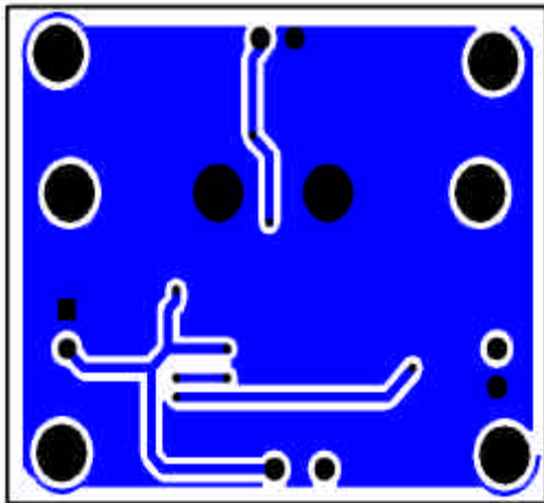
Bottom Layer
