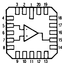
20-Pad LCC
