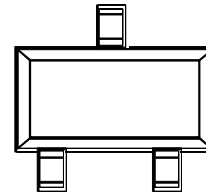
SOT-323
