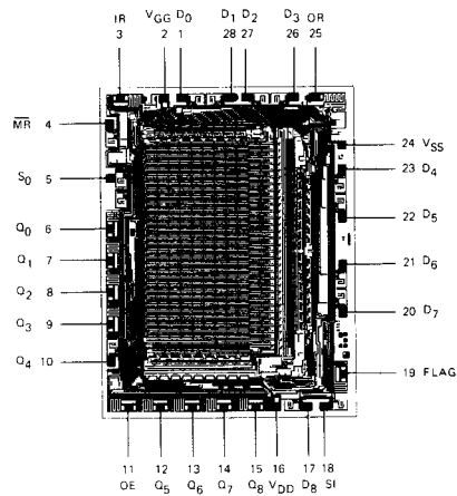
Am2813
