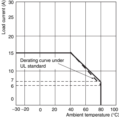
G3PB-215B-3N-VD G3PB-215B-2N-VD
