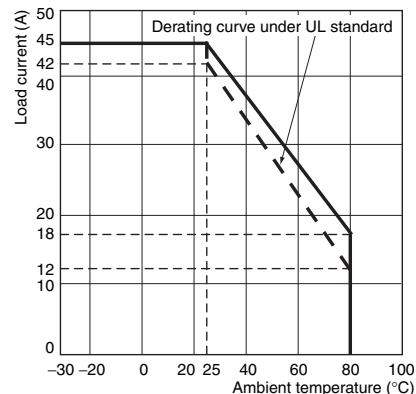
G3PB-545B-3N-VD G3PB-545B-2N-VD
