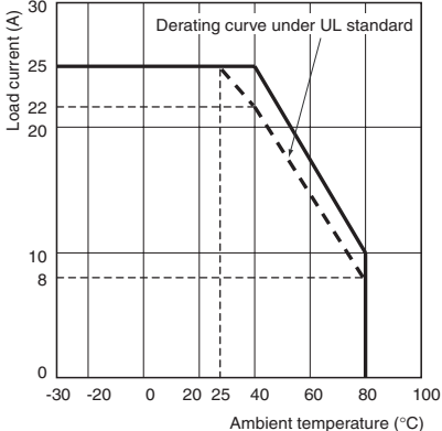
G3PB-225B-3N-VD G3PB-225B-2N-VD
