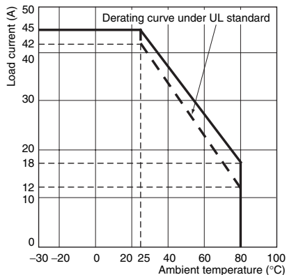
G3PB-245B-3N-VD G3PB-245B-2N-VD
