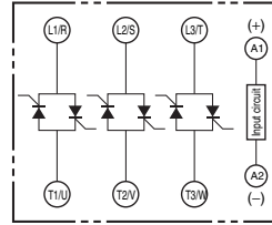
G3PB-535B-3N-VD
