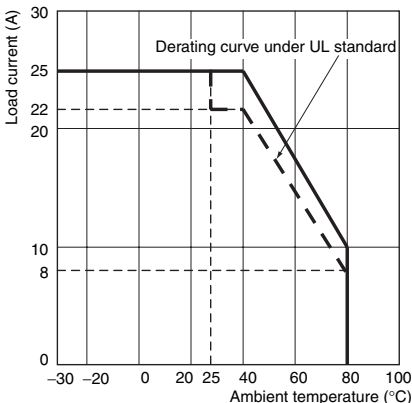
G3PB-525B-3N-VD G3PB-525B-2N-VD
