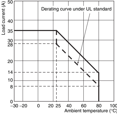
G3PB-235B-3N-VD G3PB-235B-2N-VD
