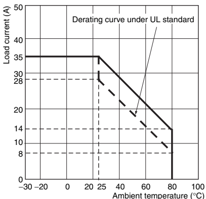
G3PB-535B-3N-VD G3PB-535B-2N-VD
