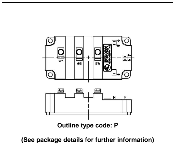
Fig. 2 Module Outline
