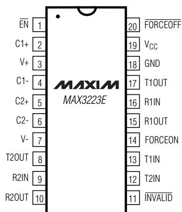
DIP/SSOP/TSSOP
