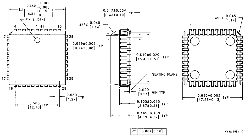
Order Number LM12454CIV, LM12458CIV, LM12H454CIV or LM12H458CIV NS Package Number V44A
