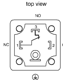
CIRCUIT DIAGRAM / Schaltbild
