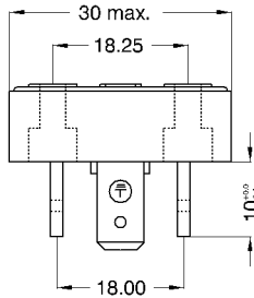
CASING / Gehäuse
