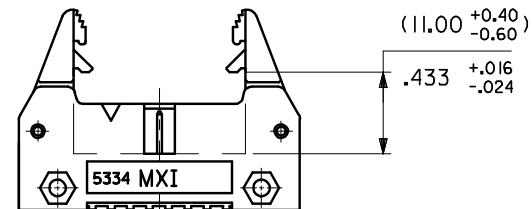
90897-1*** NON STRAIN RELIEF VERSION
