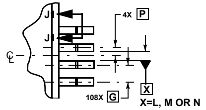
VIEW Y
