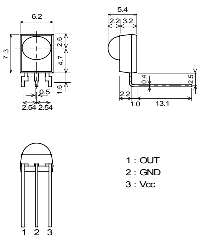
NJL21H000AF3 UNIT:mm
