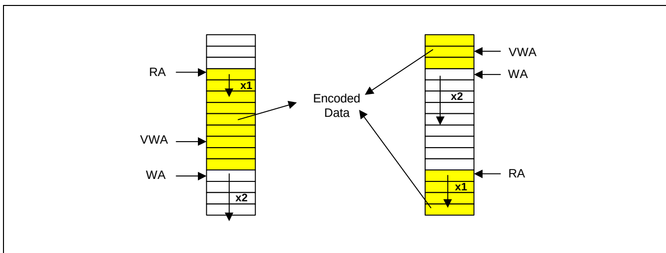
&lt;RA/WA Mapping&gt;
