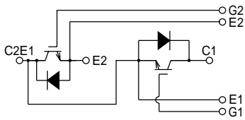
回路図 CIRCUIT
