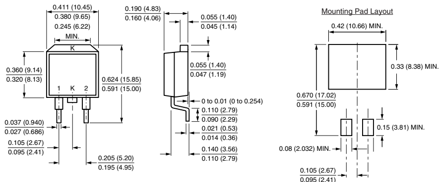
TO-263AB
