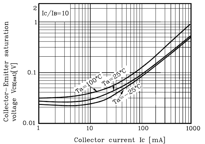
Fig. 4 V_{CE(SAT)} - I_c
