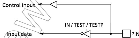
Figure 3-9. Port KE
