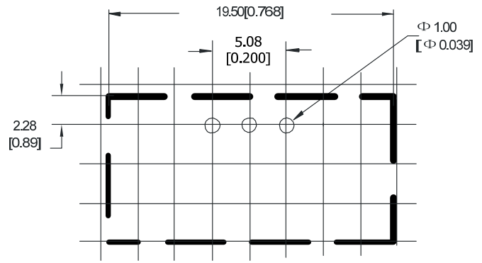
建议PCB图
