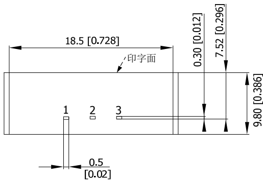
底视图
