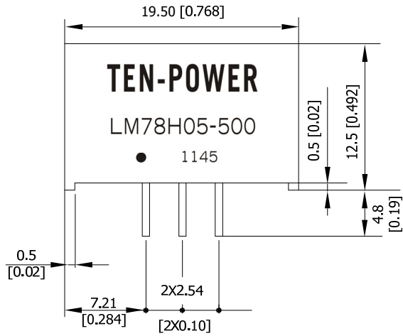
正视图
