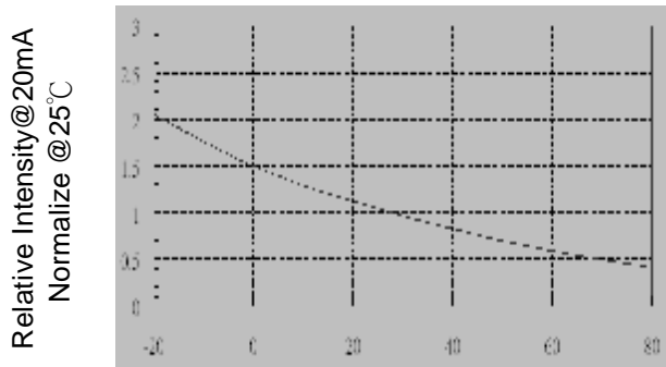
Ambient Temperature(°C)
