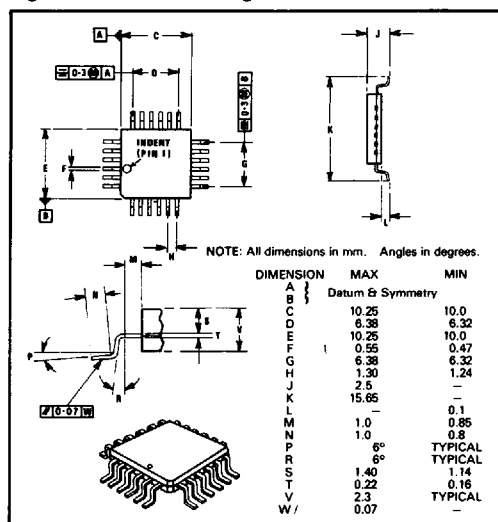
Fig. 8 FX365LS Package
