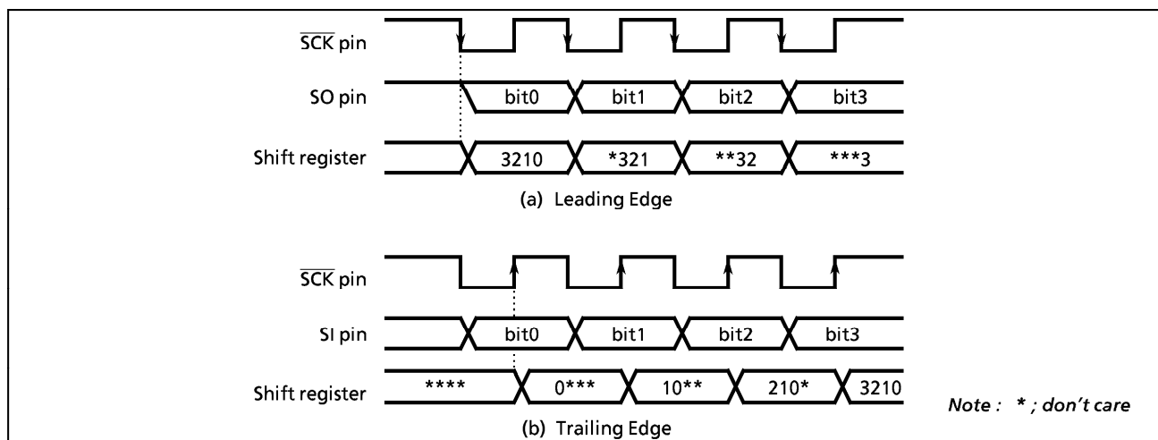
Figure 2-39. Shift Edge
