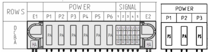
Output con.: FCI (51732-020 LF)
