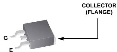
JEDEC TO-263AB
