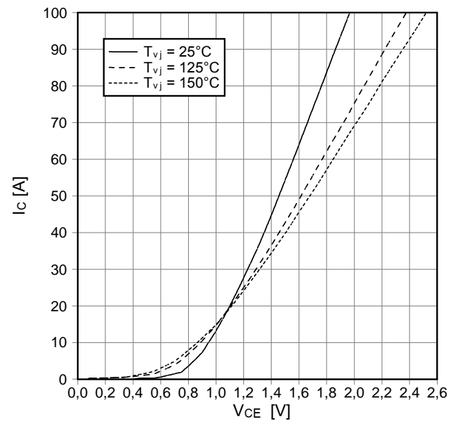
Ausgangskennlinie IGBT-Brems-Copper (typisch) output characteristic IGBT-brake-chopper (typical) I_C = f(V_{CE}) V_{GE} = 15\text{ V}
