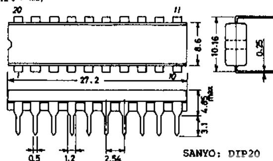
外形図 3008A-D20IC (unit: mm)
