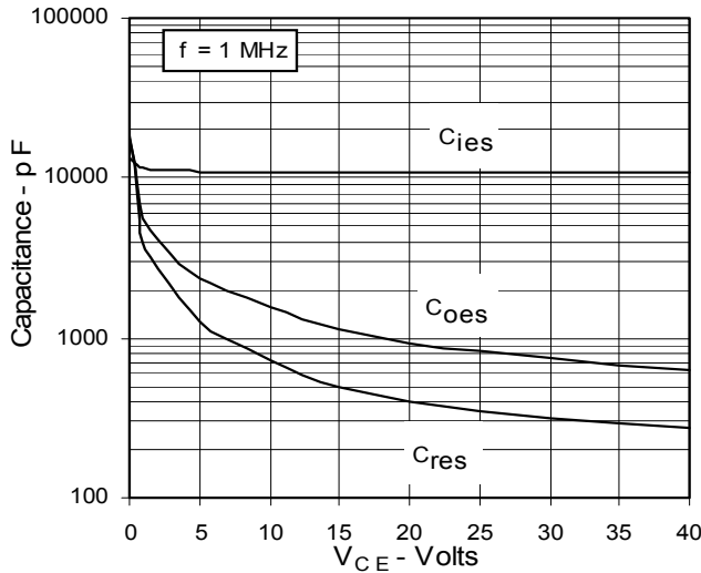
Fig. 15. Capacitance
