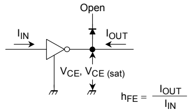
2. V_{CE(sat)} , h_{FE}
