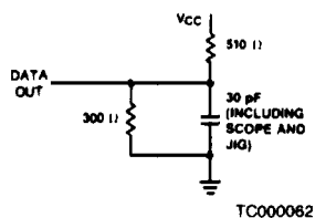
A. Output Load
