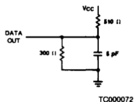
B. Output Load for t_{HZ} , t_{LZ} , t_{OW} , t_{WZ}
