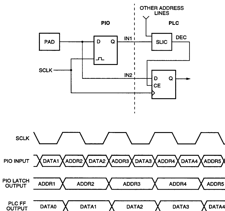
Figure 24. PIO Input Demultiplexing
