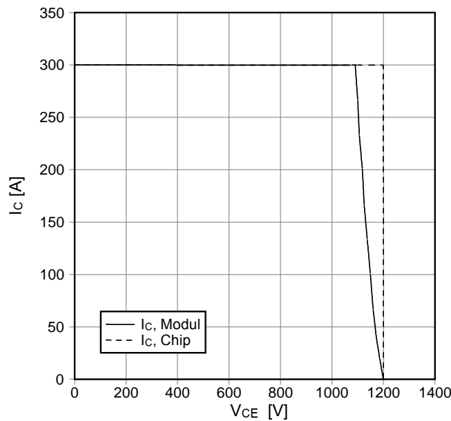
Sicherer Rückwärts-Arbeitsbereich IGBT-Wr. (RBSOA) reverse bias safe operating area IGBT-inv. (RBSOA) I_C = f(V_{CE}) V_{GE} = \pm 15\text{ V} , R_{Goff} = 8,2\ \Omega , T_{vj} = 125^\circ\text{C}
