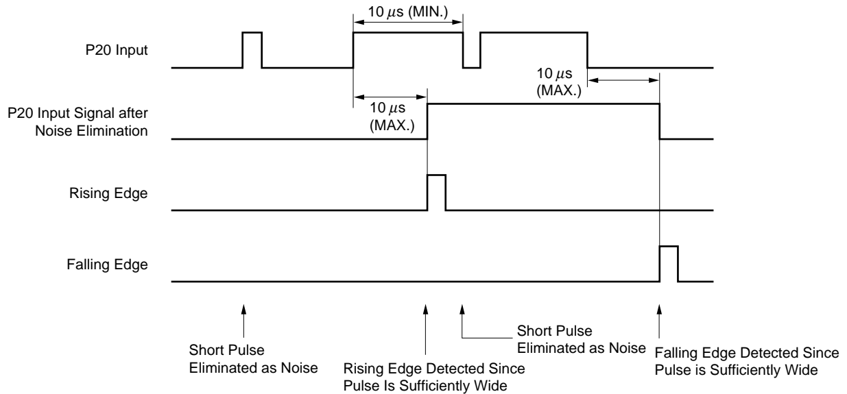
Figure 15-6. Edge Detection for Pin P20
