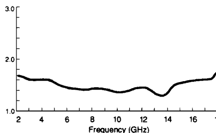
VSWR
