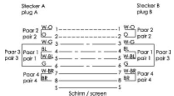
Schaltbild / Connection Diagram
