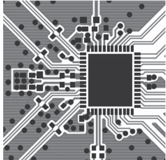
Top Side
