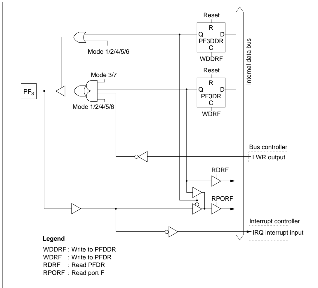
Figure C.10 (d) Port F Block Diagram (Pin PF 3 )
