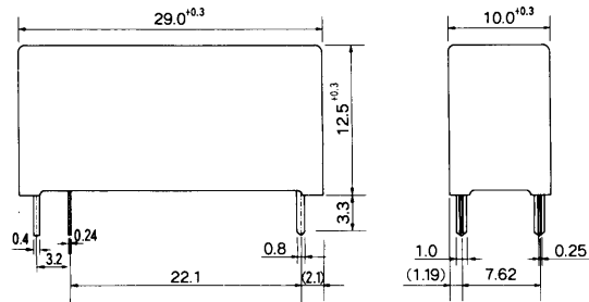
JS-K type
