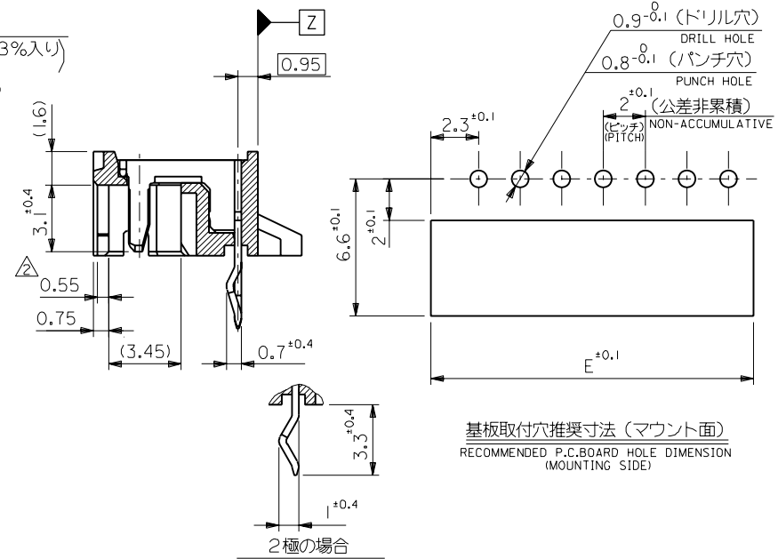
2極の場合 IN CASE OF 2 CIRCUIT
