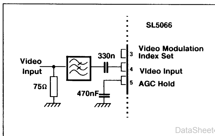
Fig.6 Video input
