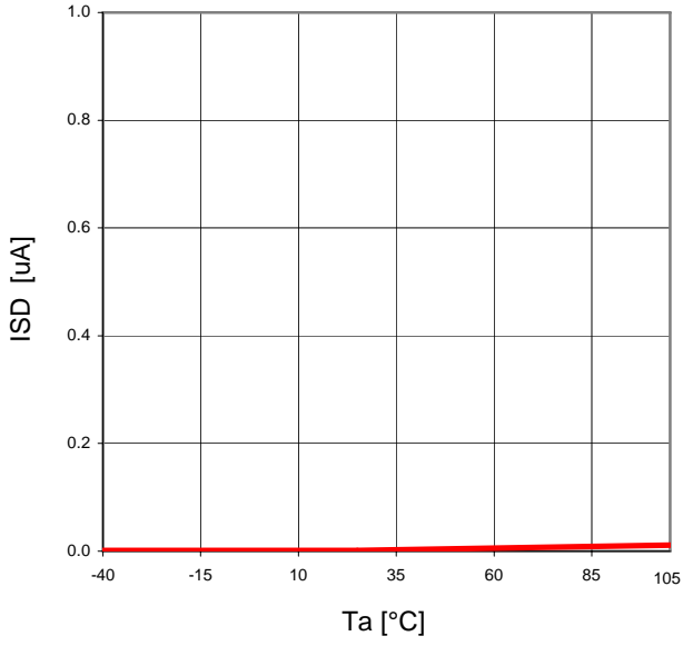
Fig.23 Ta-ISD (VEN=0V)
