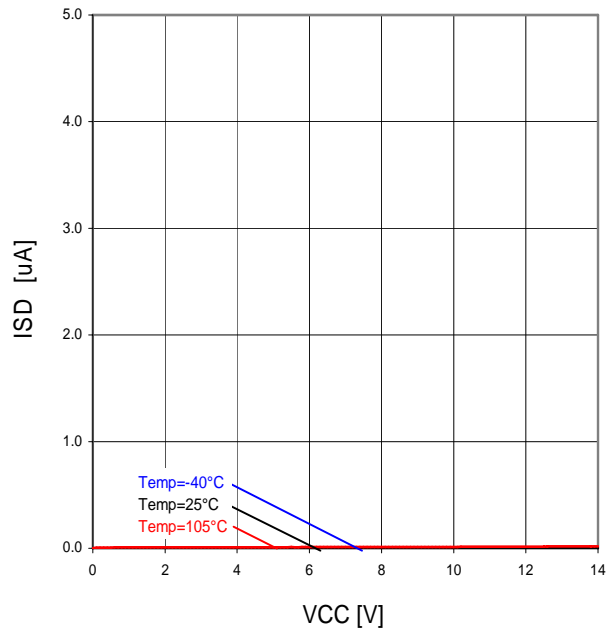
Fig.26 VCC-ISD (VEN=0V)
