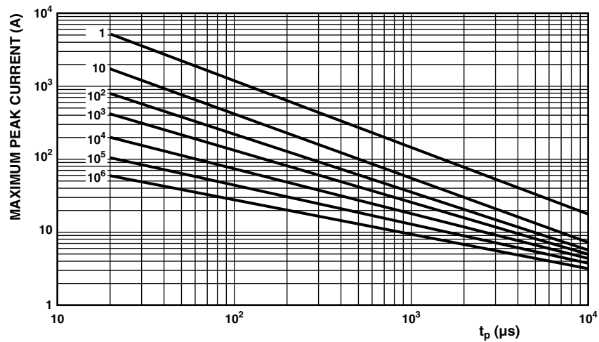
11 V RMS to 40 V RMS ; VDRH20.....E
