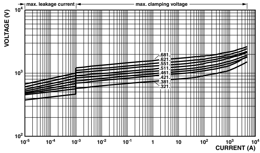
11 V RMS to 40 V RMS ; VDRH20.....E
